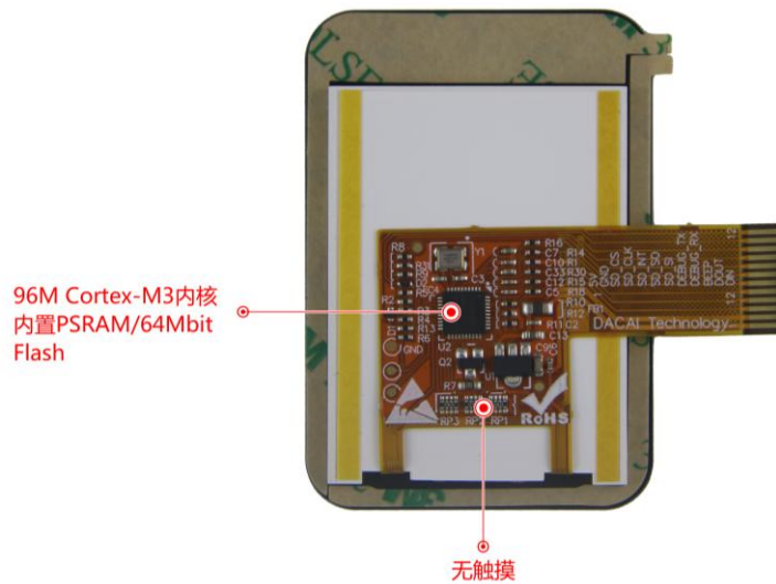
图 1-2 硬件配置图
