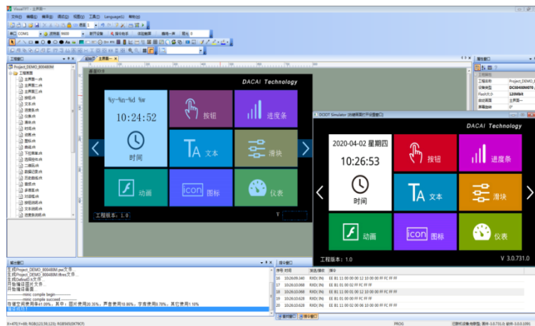
图 8-1 VisualTFT 主界面
